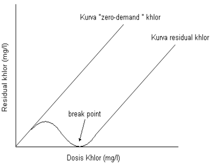
Gambar 3.34 : Kurva Kebutuhan Dosis Untuk Reaksi Khlorin Dengan Amonia.
