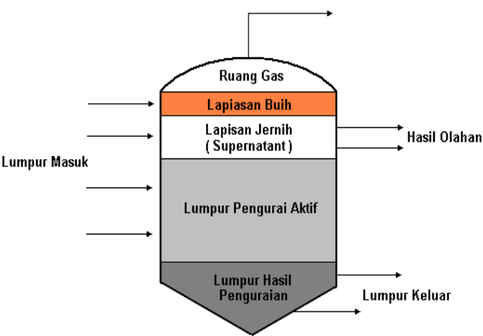
Gambar 2.4 : Penguraian Anaerob Satu Tahap.
