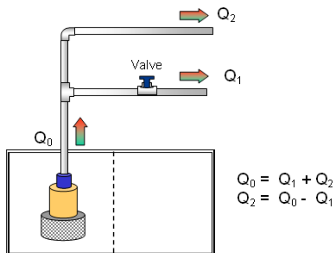
Gambar 4.1 : Diagram Pompa Air Limbah Dengan Valve By Pass.
