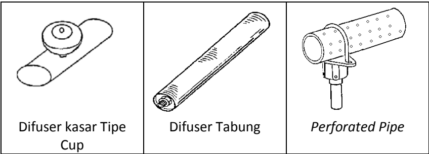
Gambar 3.26 : Beberapa Contoh Tipe Aerator Dan Difuser.
