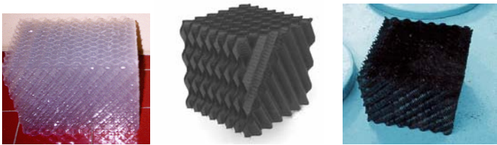
Gambar 2.14 : Bentuk Media Terstruktur Tipe Sarang Tawon ( Cross Flow ) Yang Banyak Digunakan Untuk Biofilter.
