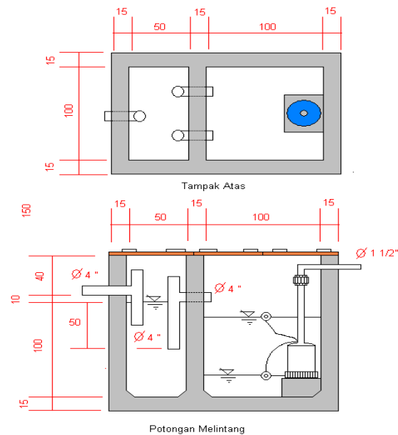
Gambar 3.3 : Salah Satu Contoh Tipikal Konstruksi Bak Pengumpul.
