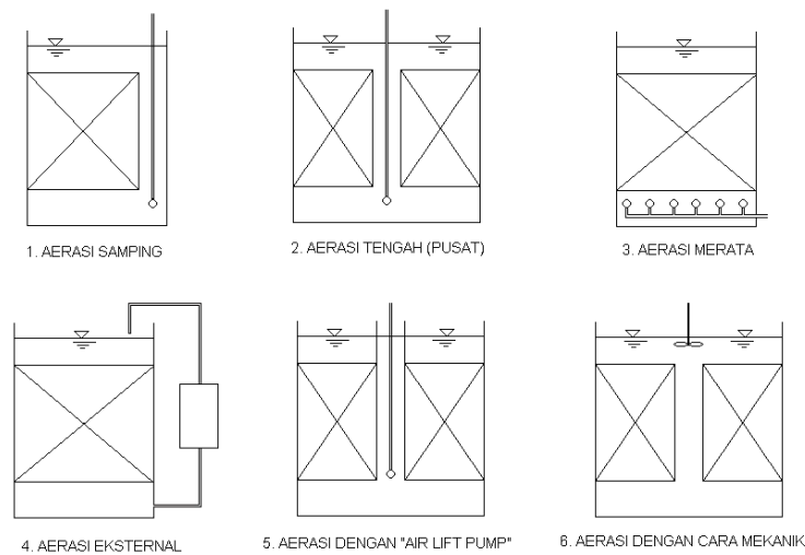
Gambar 2.3 : Beberapa Metoda Aerasi Untuk Proses Pengolahan Air Limbah Dengan Sistem Biofilter Tercelup.
